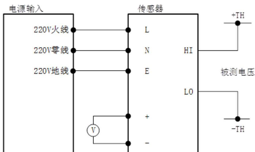
图 3 电气连接图
