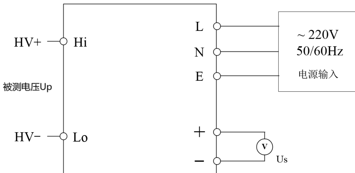
图 3 电气连接图
