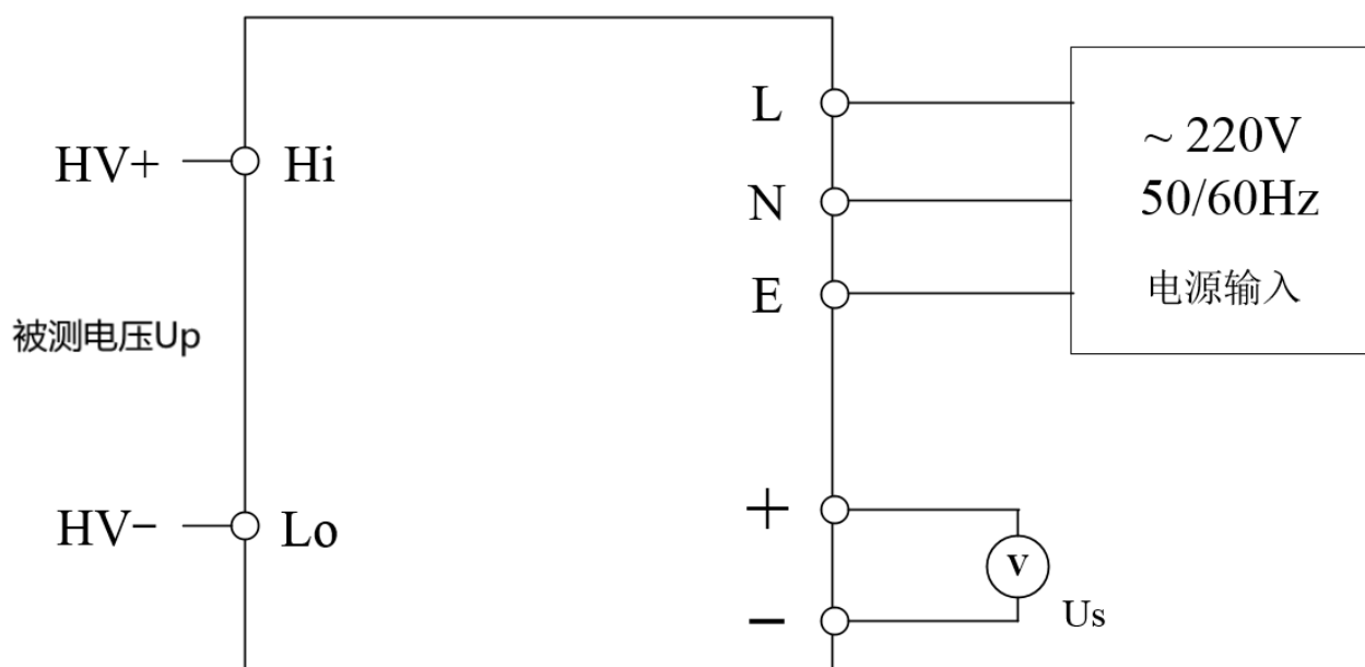
图 3 电气连接图
