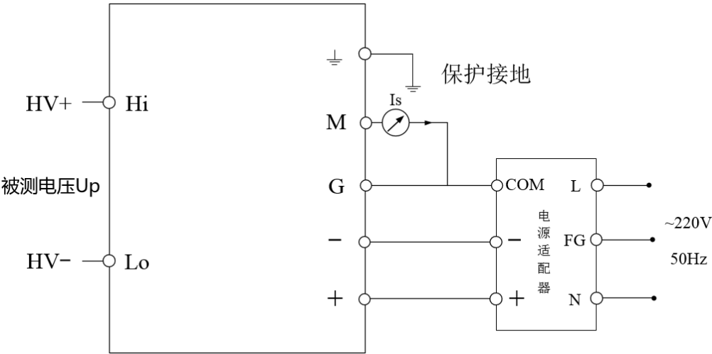
图 3 电气连接图
