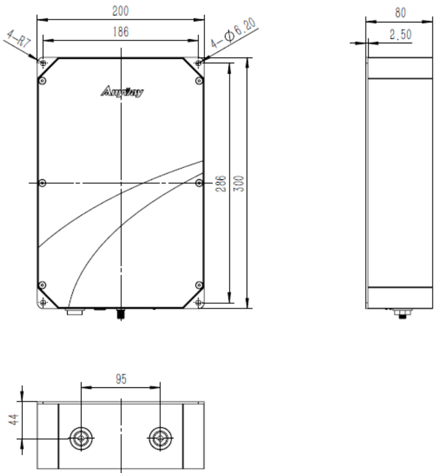
图 1 外形尺寸图
