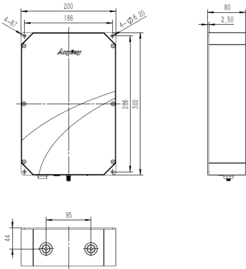
图 1 外形尺寸图
