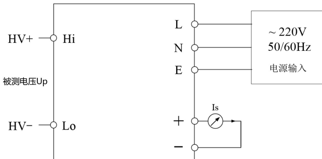
图 3 电气连接图
