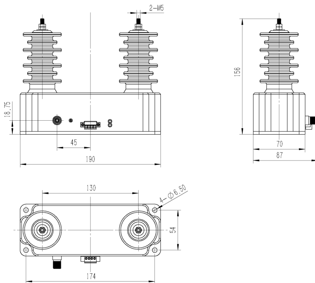
图 1 外形尺寸图
