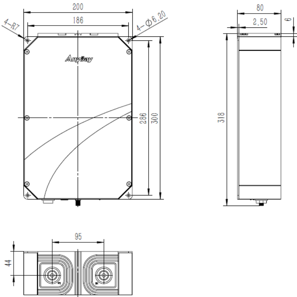
图 1 外形尺寸图
