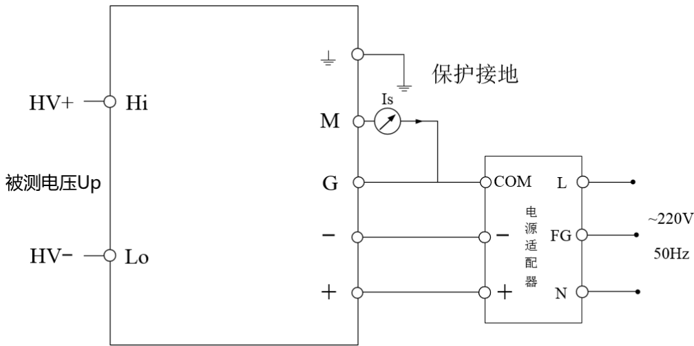
图 3 电气连接图
