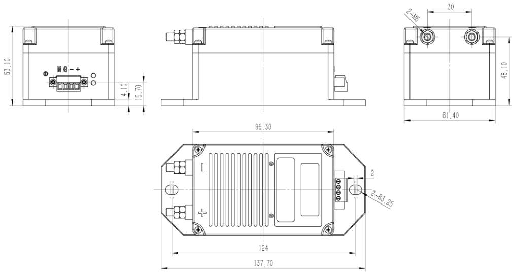
图 1 外形尺寸图
